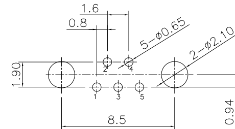
P.C.B Layout \triangle E
